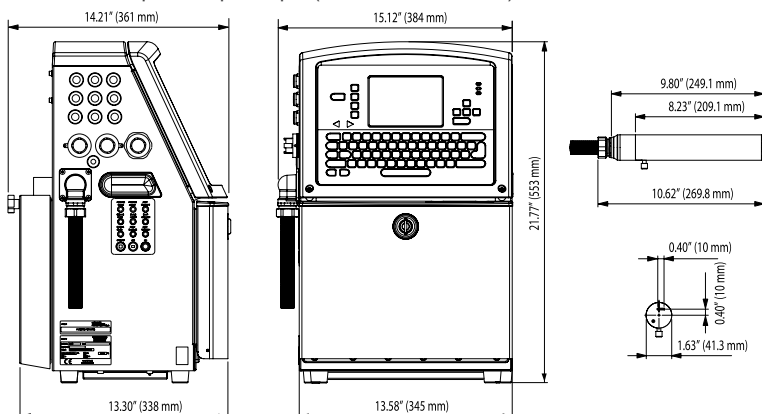
Габаритные размеры (класс защиты IP65)
